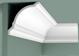
CX203 200 x 14,5 x 14,5 cm Duropolymer®
