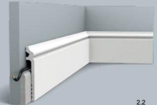
SX186 CONTOUR 200 x 13,8 x 2,2 cm Duropolymer®
