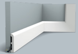
SX183 | SX183F CASCADE SX183-RAL9003 200 x 7,5 x 1,3 cm Duropolymer®
