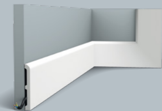
SX184 | SX184F CASCADE 200 x 11 x 1,3 cm Duropolymer®
